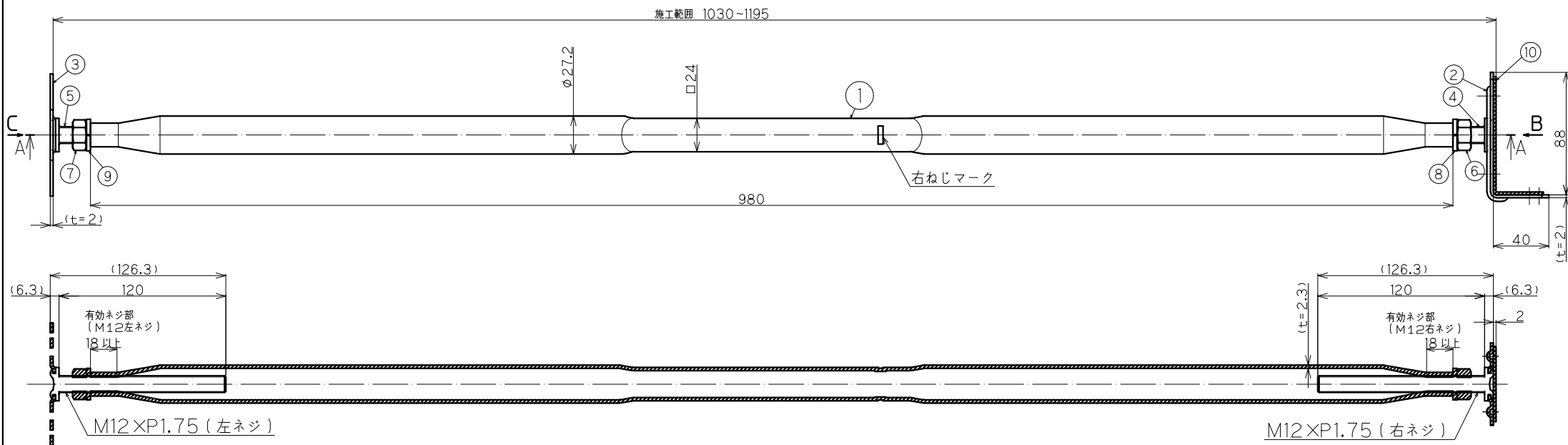
A-A断面図
