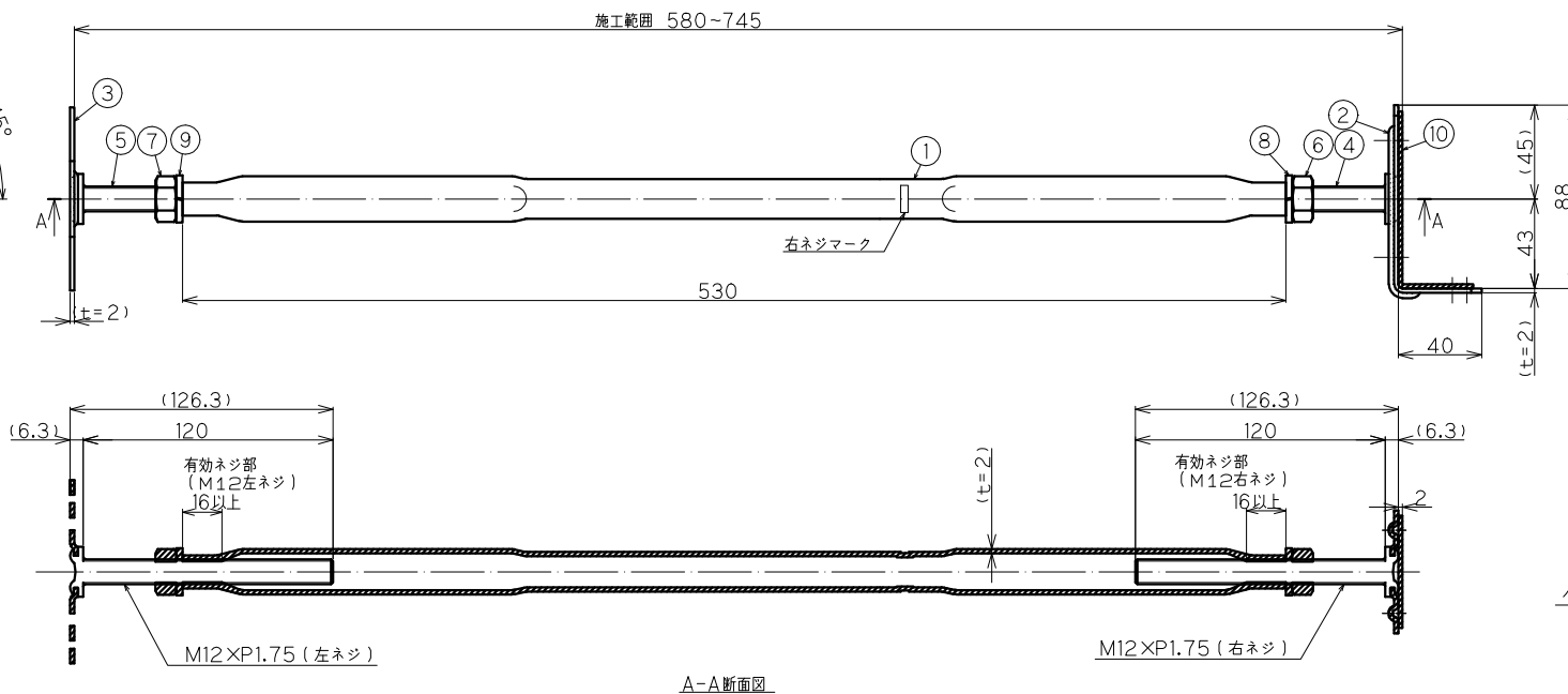
A-A断面図
