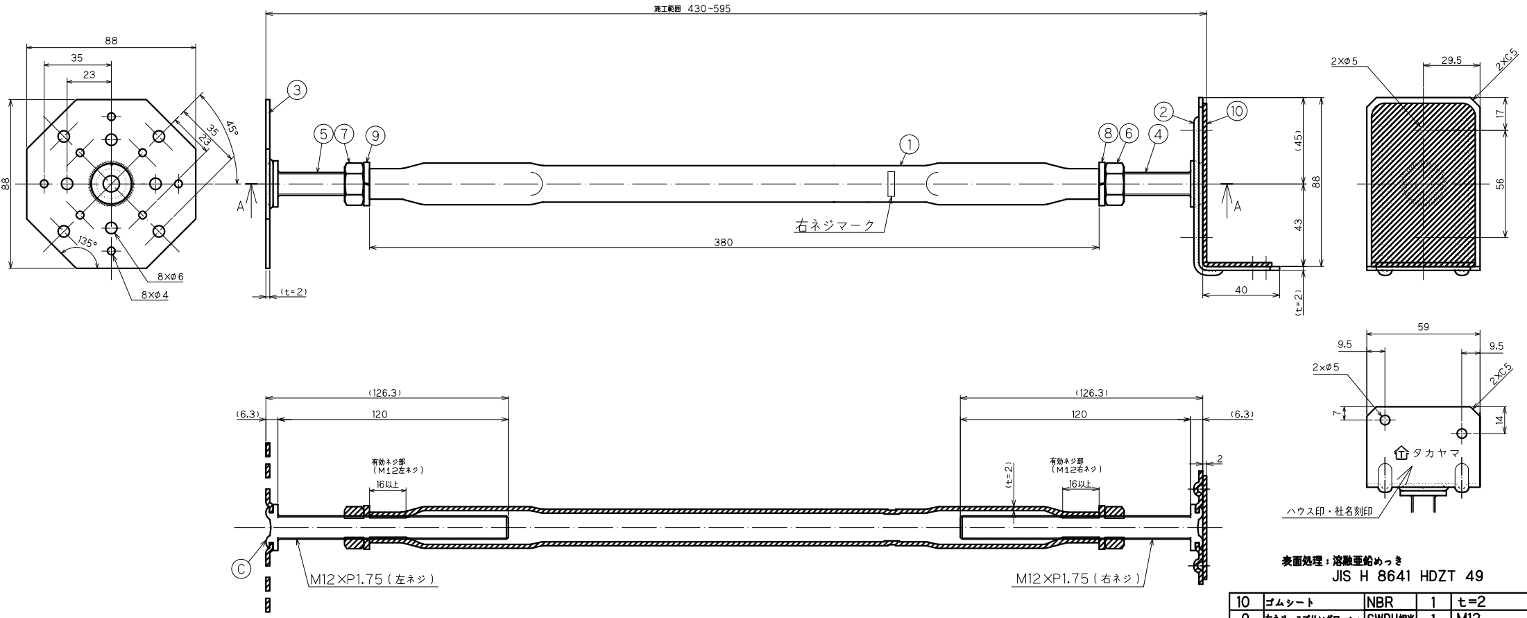
A-A断面図
