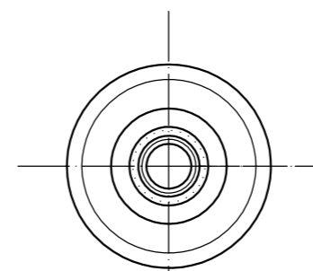
カシメナット取付状態 (フェルト貼り付け前)
