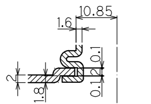
パイプカシメ部断面詳細 S=2/1
