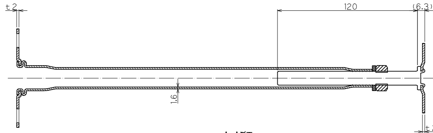
A-A断面
