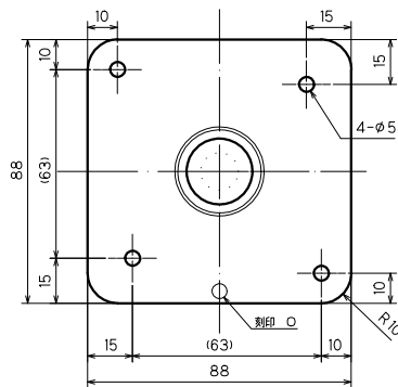
矢 視 B
