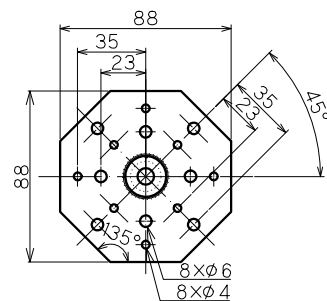
矢視C
