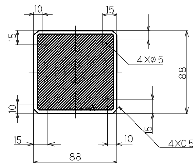
矢視B
