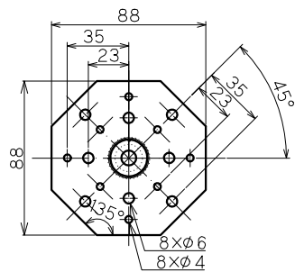
矢視C
