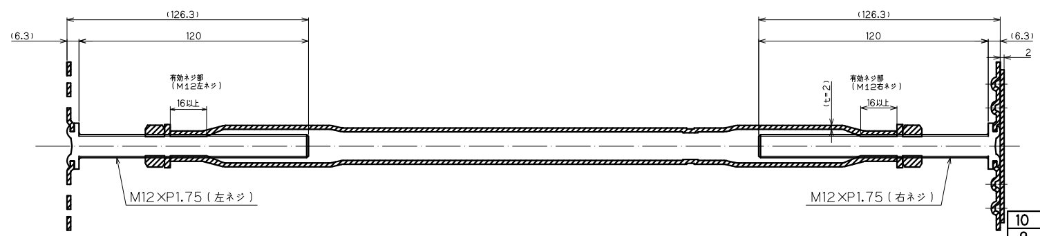
A-A断面図
