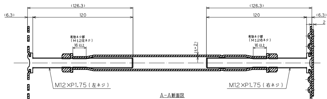
A-A断面図
